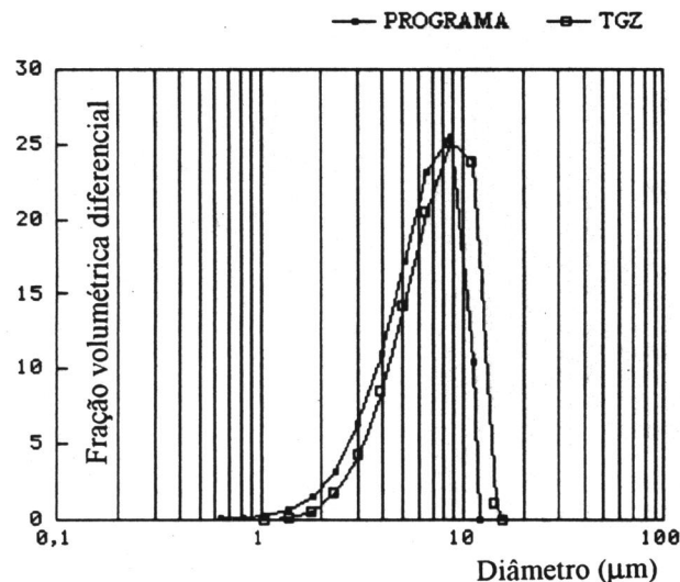
Figura 5: Distribuições de tamanhos de grão Óxido de urânio e estearato
