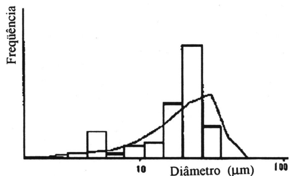
Figura 2: Distribuições de tamanhos Computador (histograma), Saltykov (polígono)
