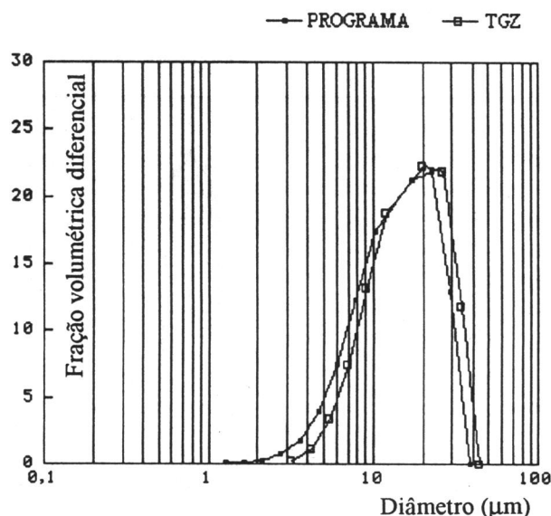
Figura 3: Distribuições de tamanhos de grão Óxido de cromo
