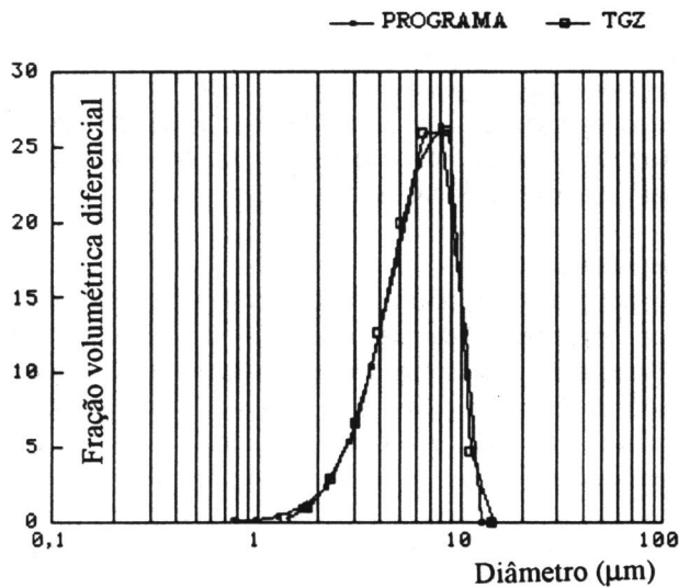
Figura 4: Distribuições de tamanhos de grão Óxido de urânio e lama de retífica
